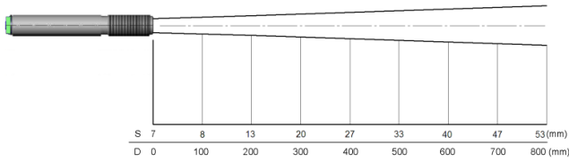
Optical chart: CS (15:1)
